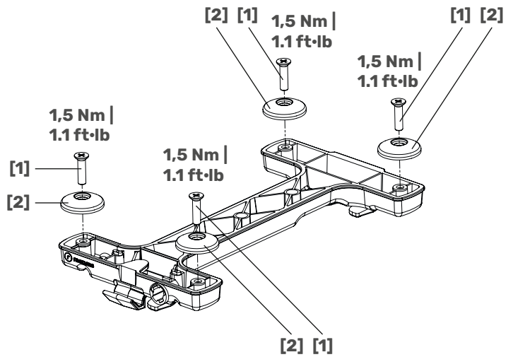
ART. 27001 | ART. 27021 Ohne Füße | Without feet | Sans pieds | Zonder voetjes | Sin patas | Senza piedini
