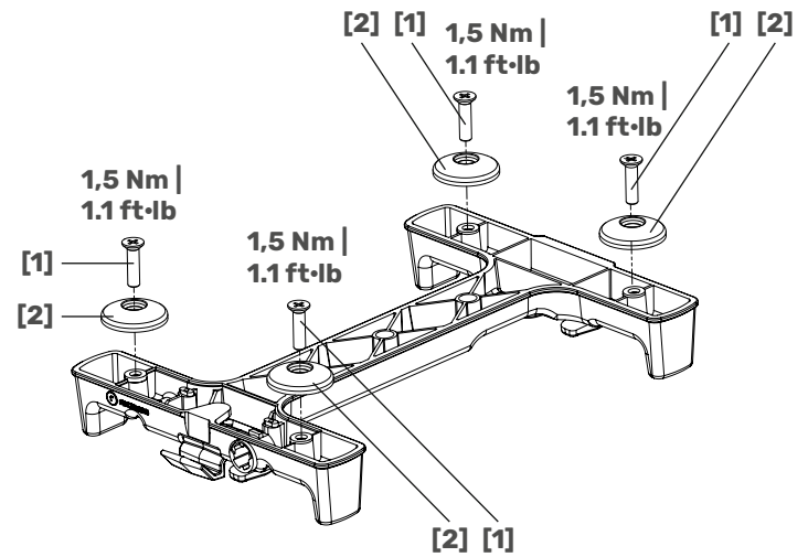
ART. 27002 | ART. 27022 Mit Füßen | With feet | Avec pieds | Met voetjes | Con patas | Con piedini
